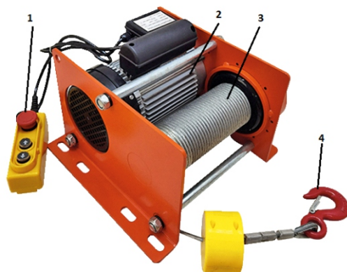
Рисунок 1. Конструкция лебедки
