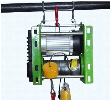
Рисунок 2. Крепление лебедки в вертикальном положении
