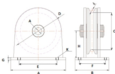
Рисунок 1. Размер блока
