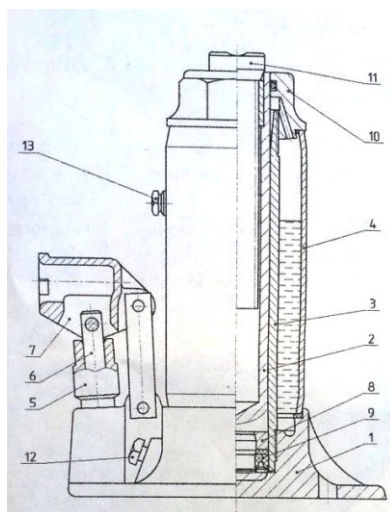
Рисунок 2. Устройство домкрата.
