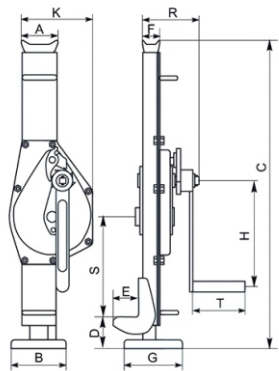
Рисунок 1. Размеры домкрата.
