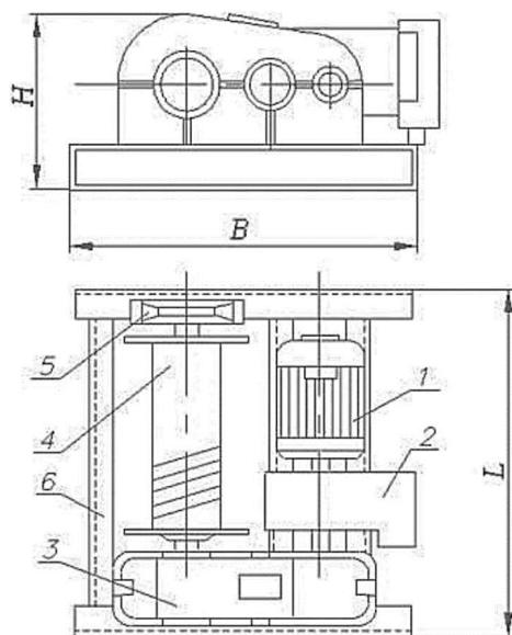
Рисунок 1. Схема лебедки ЛМ.
