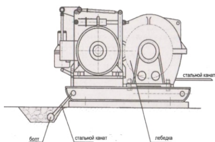
Рисунок 5.Крепление стальным канатом.
