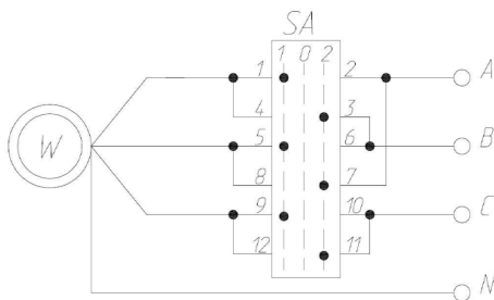
Рисунок 4.1 Электрическая схема лебедки JM, г/п 0,5-5т.
