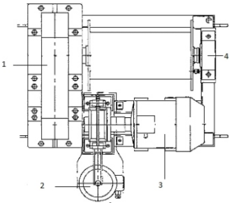
Рисунок 7. Схема мест смазывания.
