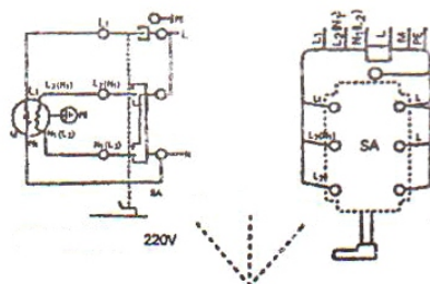
Рисунок 4. Схема подключения электролебедки 220В.
