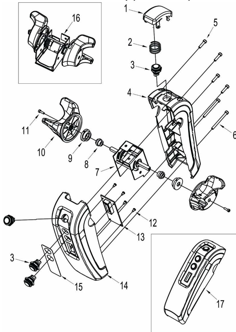
Схема 2. Блок управления в сборе.
