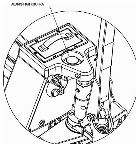
Рисунок 5. Кнопка аварийной остановки
