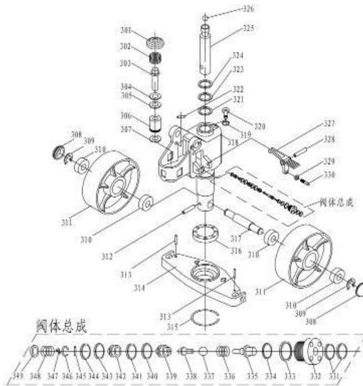
Рисунок 7. Взрыв-схема гидроузла тележки BFL
